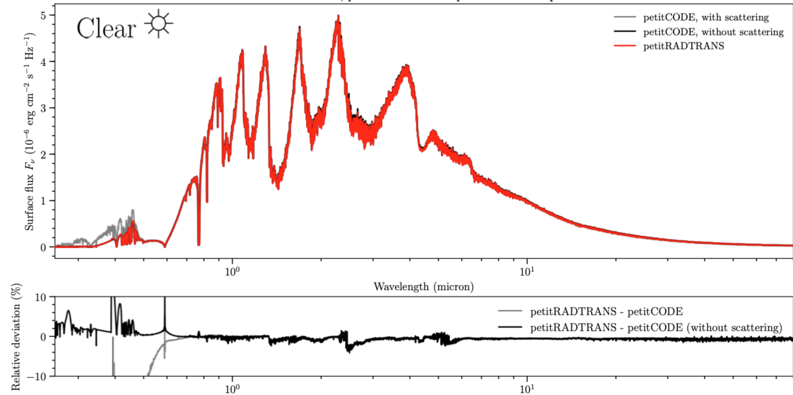
Clear TrES-4b, petitRADTRANS – petitCODE comparison
